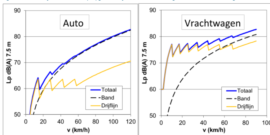
Figuur 2. Aandrijf- en banden(rol)geluid bij auto's/vrachtwagens met verbrandingsmotor. 28
