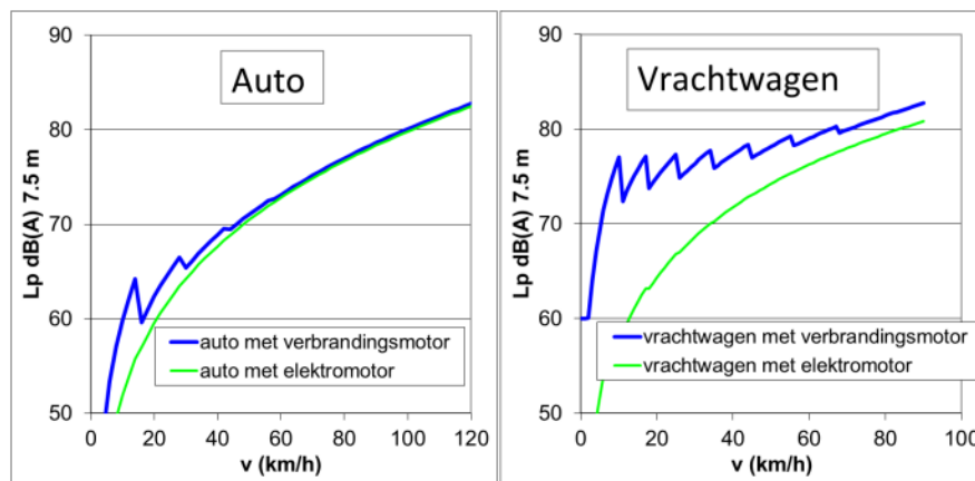
Figuur 3. Aandrijf- en banden(rol)geluid verbrandingsmotor versus elektromotor. 30
